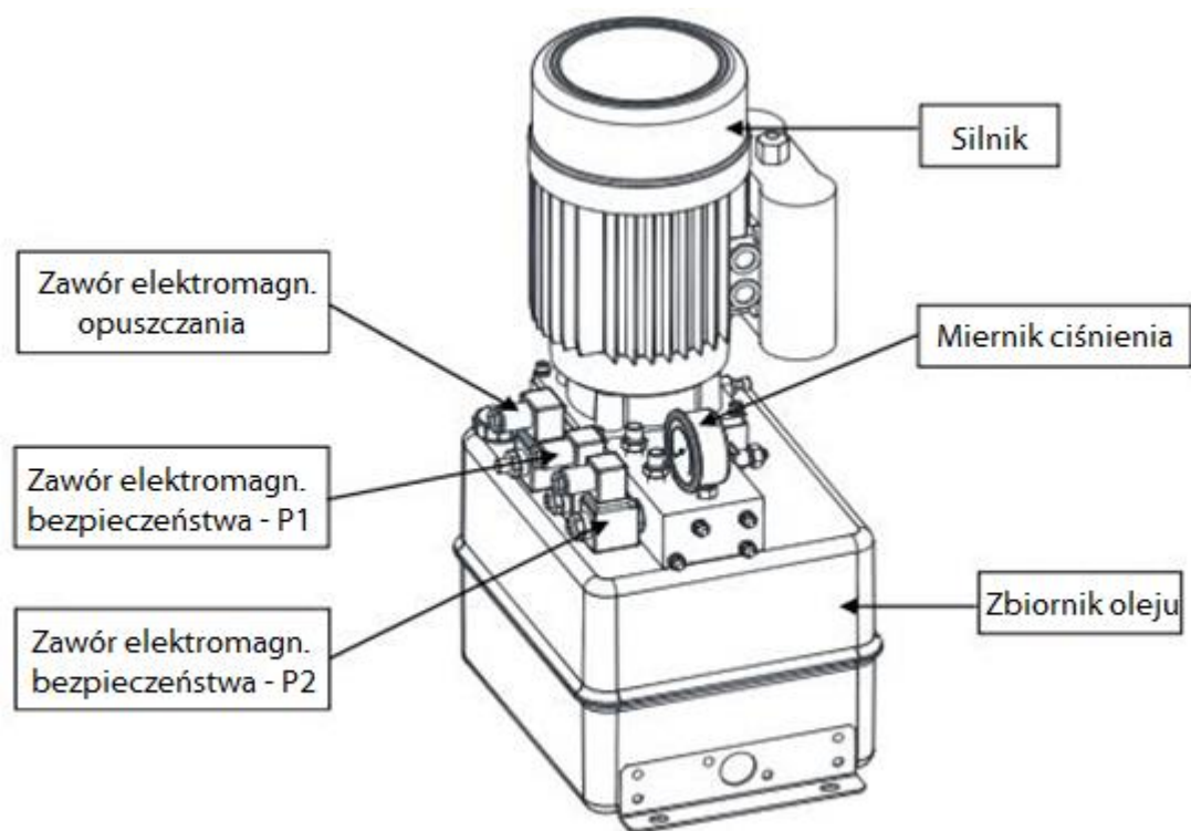
Rysunek 3 – HYDRAULICZNY ZESPÓŁ NAPĘDOWY
