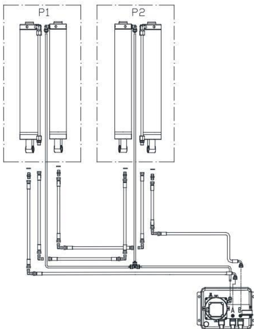
Rysunek 12 – PODŁĄCZENIE HYDRAULICZNE
